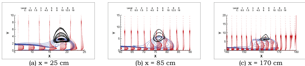
圖 15 C_{in}=17.17 g/L, Q_{in}=2.18 L/min 之異重流頭端流速向量圖
