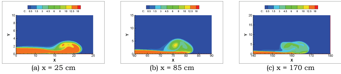
圖 10 C_{in}=17.17 g/L, Q_{in}=2.18 L/min 之異重流頭端數值濃度分佈
