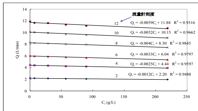
圖 4 鹽水流量計讀數與實際鹽水入流量迴歸關係圖
