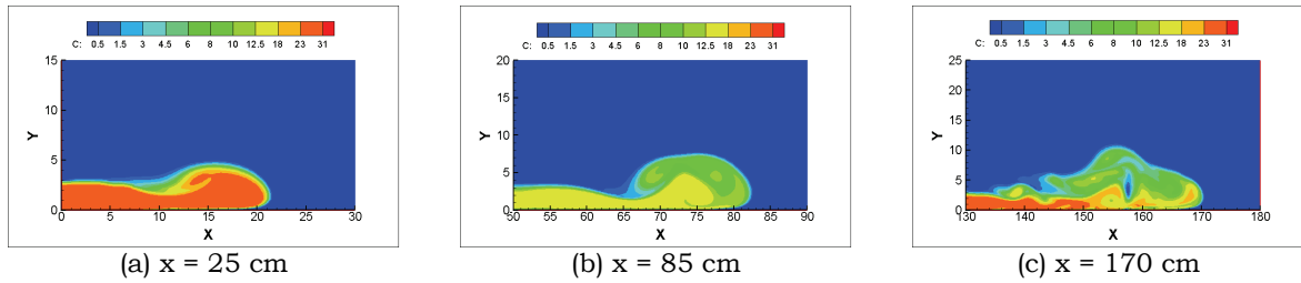
圖 12 C_{in}=30.61 g/L, Q_{in}=5.94 L/min 之異重流頭端數值濃度分佈
