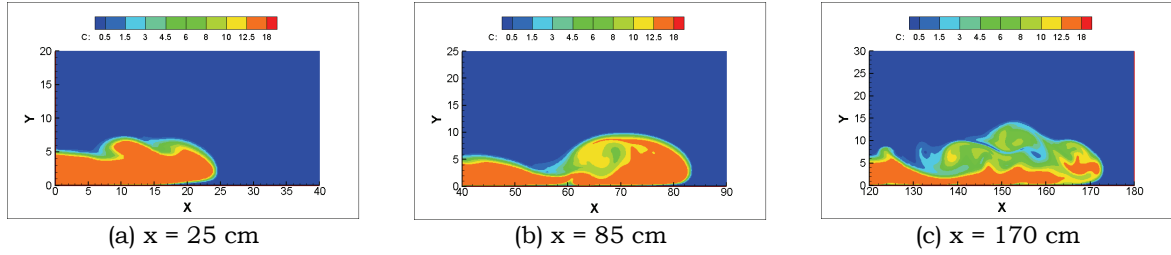
圖 11 C_{in}=17.17 g/L, Q_{in}=11.78 L/min 之異重流頭端數值濃度分佈
